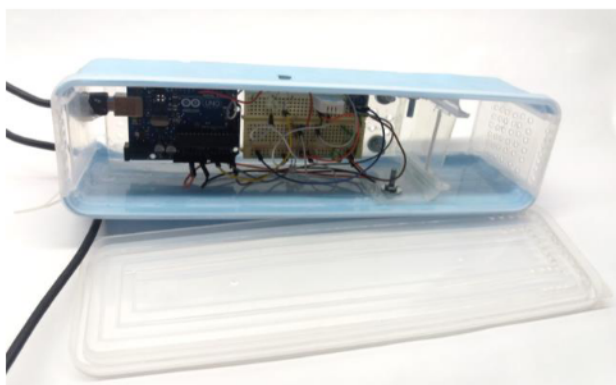
Figura 5 - Protótipo da estação meteorológica com o uso do Arduino e do Processing
