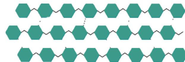
Celulose
