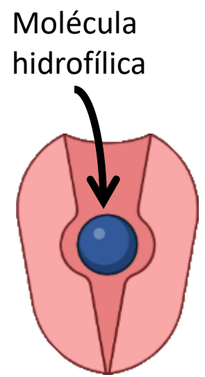
Proteína transportadora
