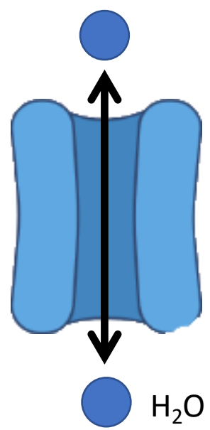
Aquaporina
