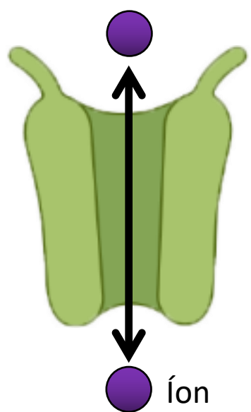
Canal iônico
